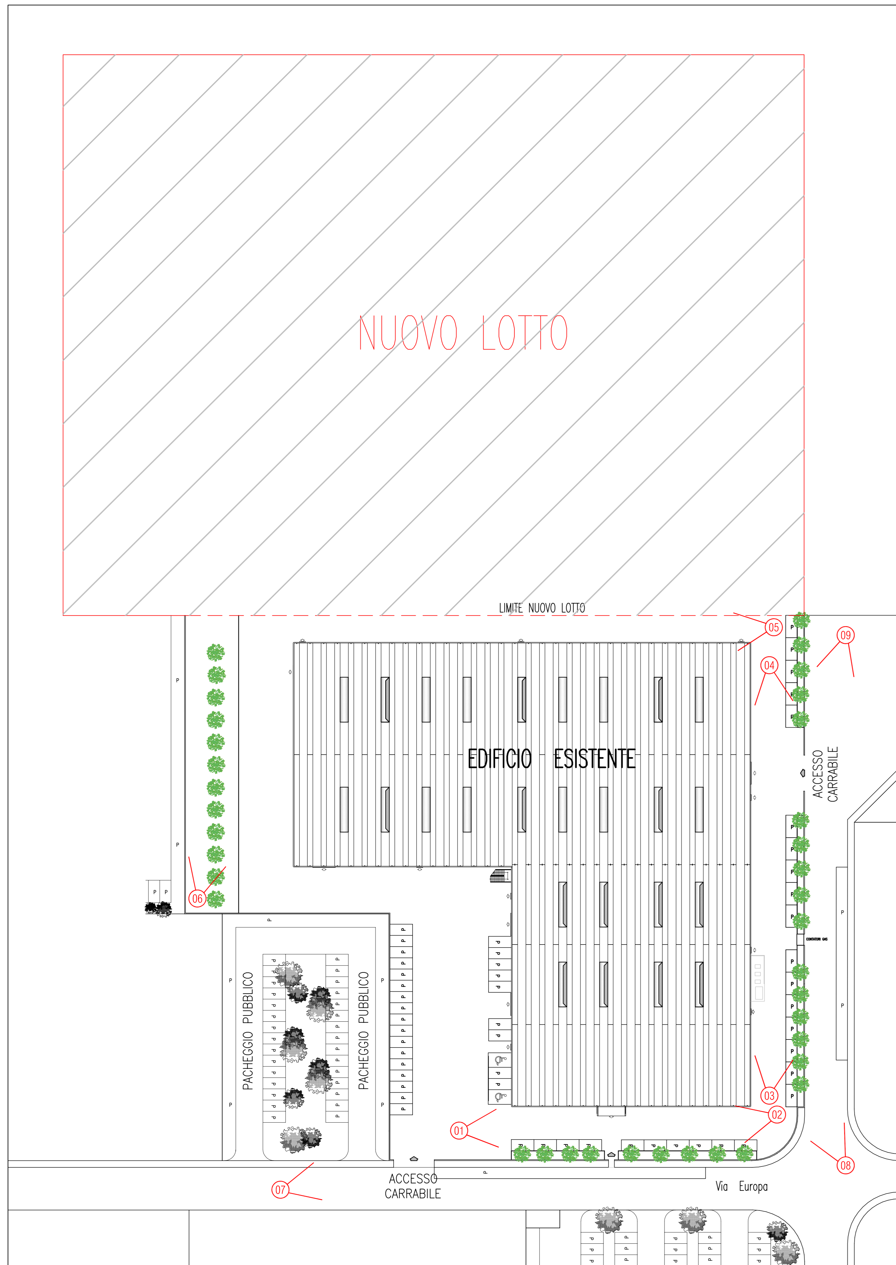
PLANIMETRIA 1 : 500
