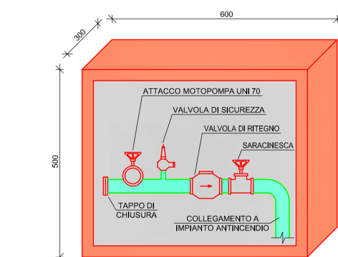
ATTACCO MOTOPOMPA IN CASSETTA CON VETRO A ROMPERE
