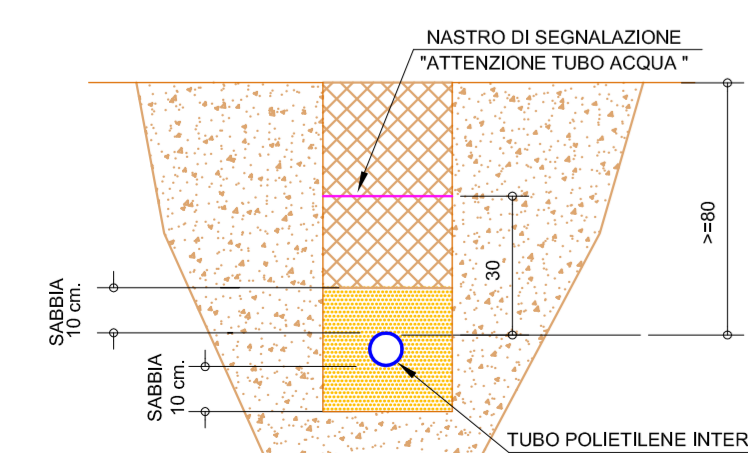
PARTICOLARE TUBO POLIETILENE INTERRATO
