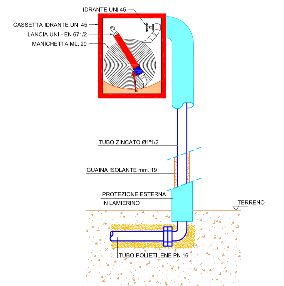
IDRANTE UNI 45
