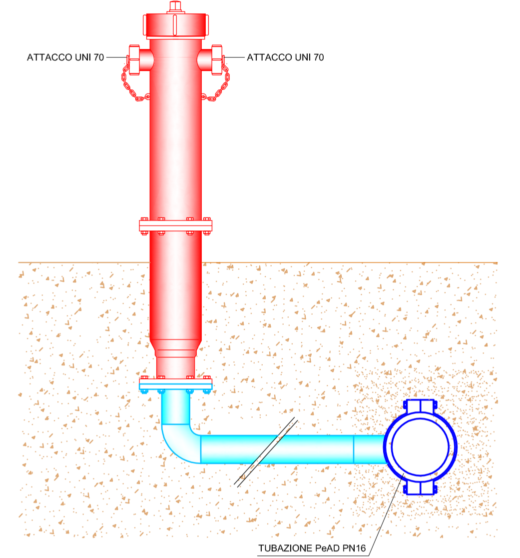
IDRANTE SOPRASSUOLO
